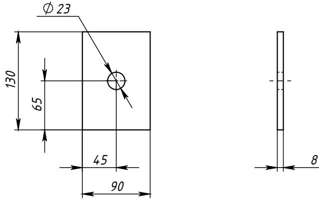
Поз.2 (Планка)
